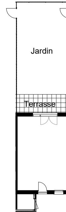
Villa n° V02 Type T4 Duplex Niveau 0 et 1 Entrée 4.19 m² Séjour / Cuisine 25.90 m² Chambre 1 9.01 m² Chambre 2 9.66 m² Chambre 3 9.20 m² Dégagement 3.09 m² Salle de bain 6.52 m² Salle d'eau 4.88 m² WC 1 1.50 m² WC 2 1.40 m² Rangement 1 2.20 m² Rangement 2 0.84 m² Surface Habitable 78.39 m² Rangement Extérieur 3.00 m² Terrasse 11.51 m² Jardin environ 52m² La surface des pièces comprend la surface des placards
