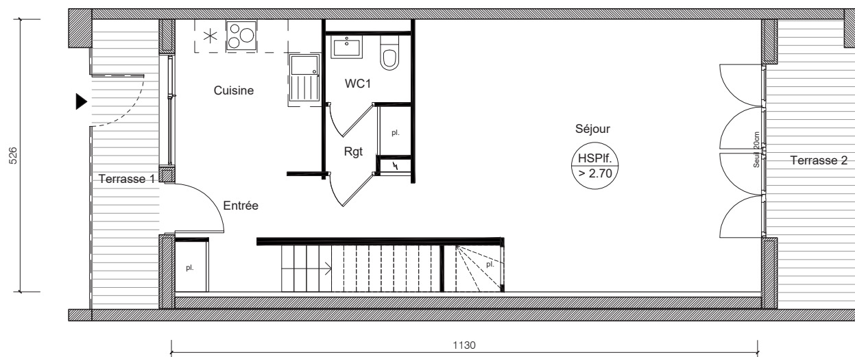
NIVEAU 0
