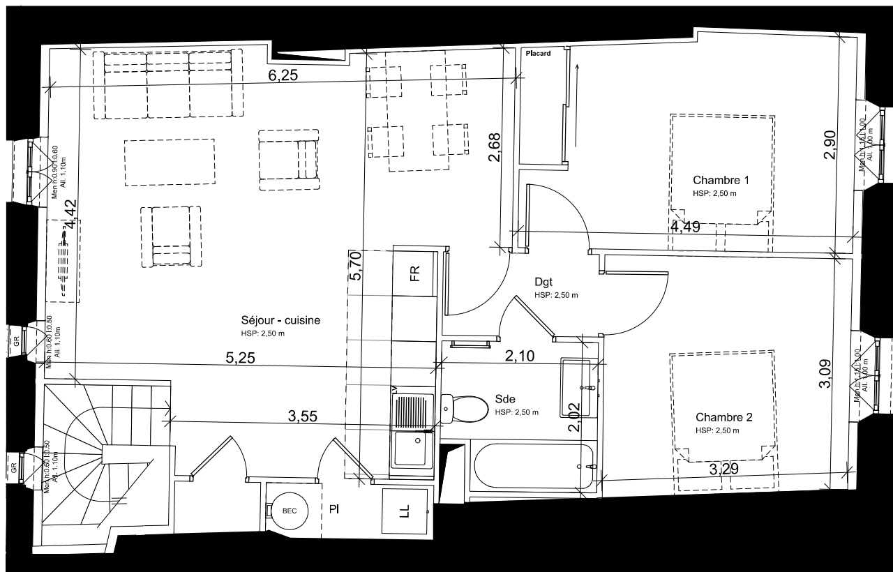
Plan R+2
