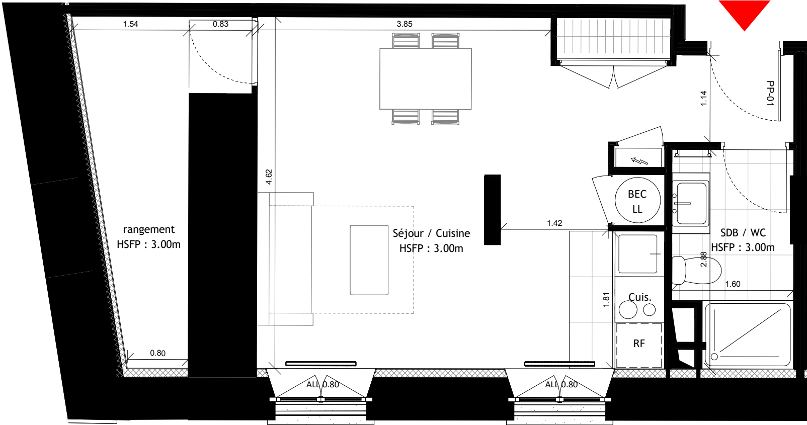
Appartement C24A Type T1
