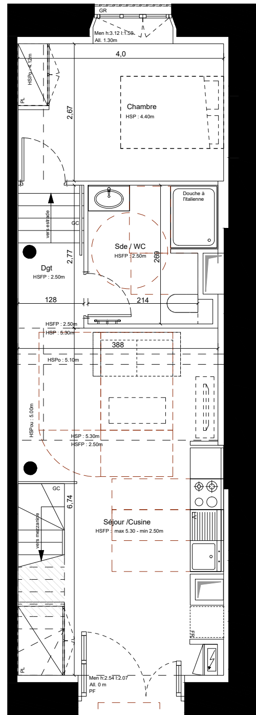
Plan RDC
