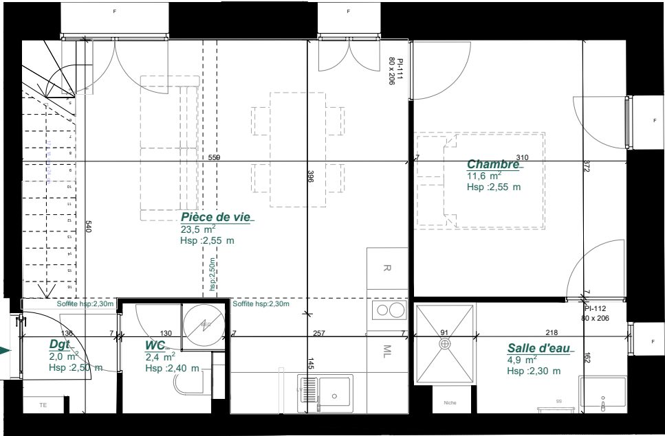
PLAN NIVEAU BAS - R+3
