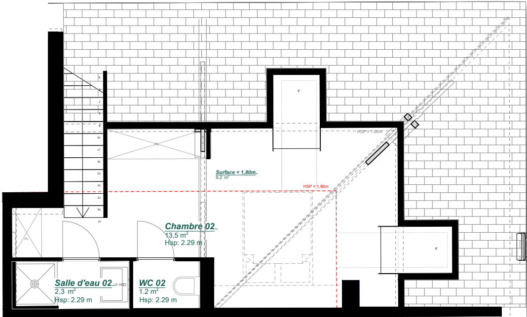
PLAN NIVEAU HAUT - R+4
