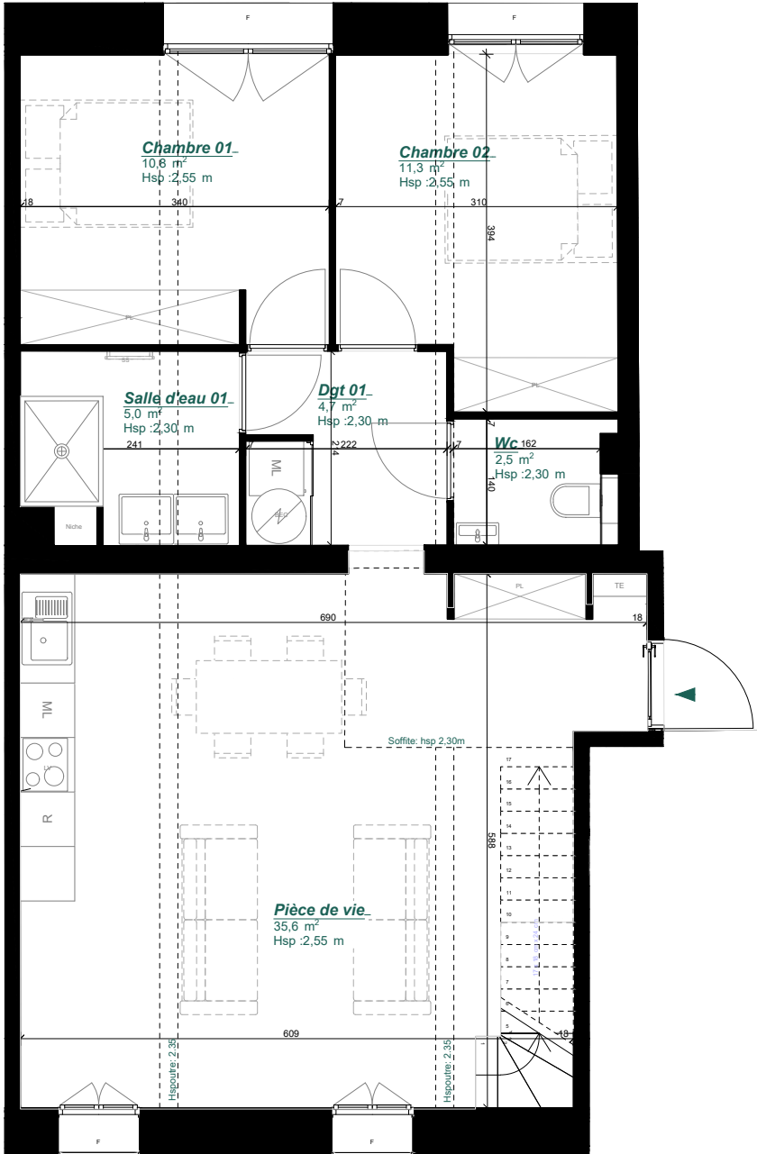
PLAN NIVEAU BAS - R+3
