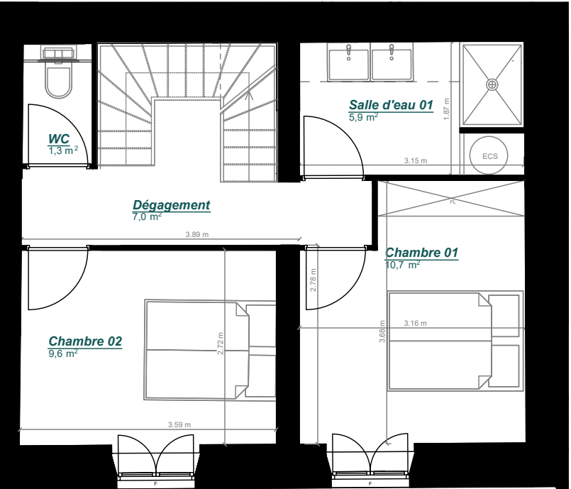
PLAN NIVEAU BAS - RDJ
