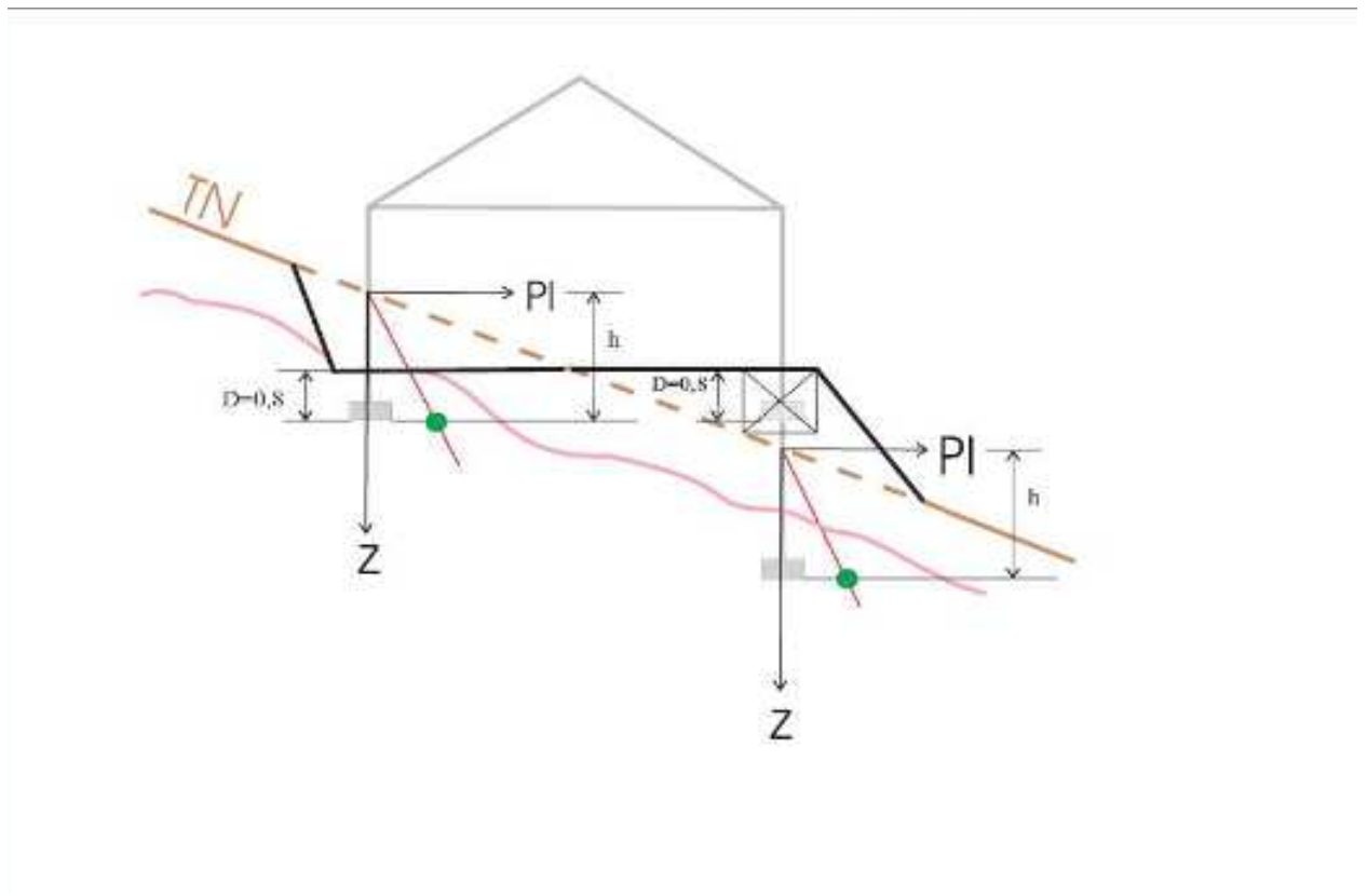
Schéma 3 : Ancrage des fondations pour des conditions mécaniques (pression limite) homogènes
