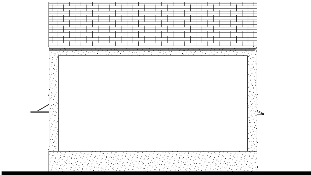
Pignon DROIT
