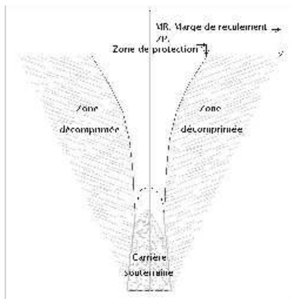
Figure 7 : Schéma zone de protection - marge de reculement
