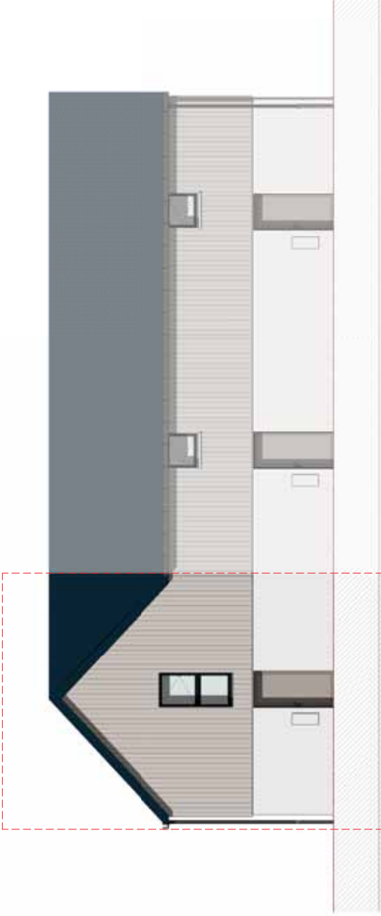
FACADE ARRIÈRE
