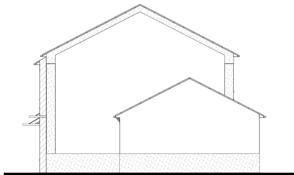
Pignon DROIT
