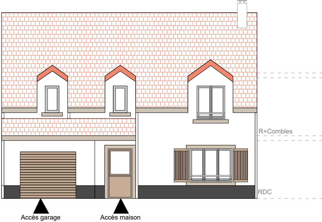
Façade AVANT
