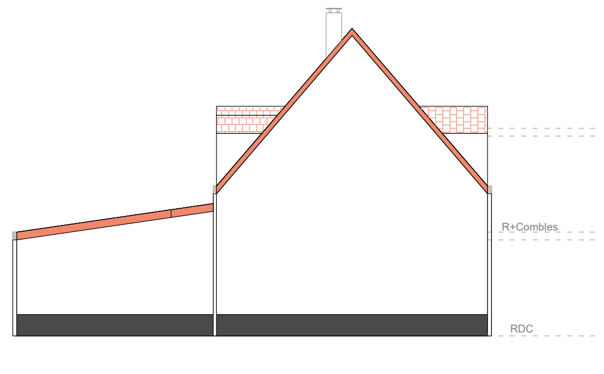
Pignon DROIT
