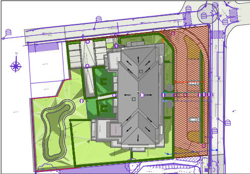
Rez de chaussée Lot A006 Type 3
