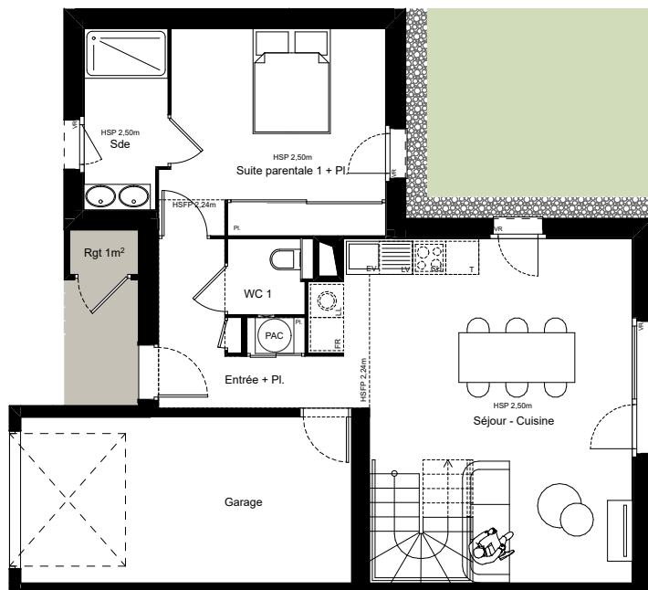
NIVEAU INFÉRIEUR
