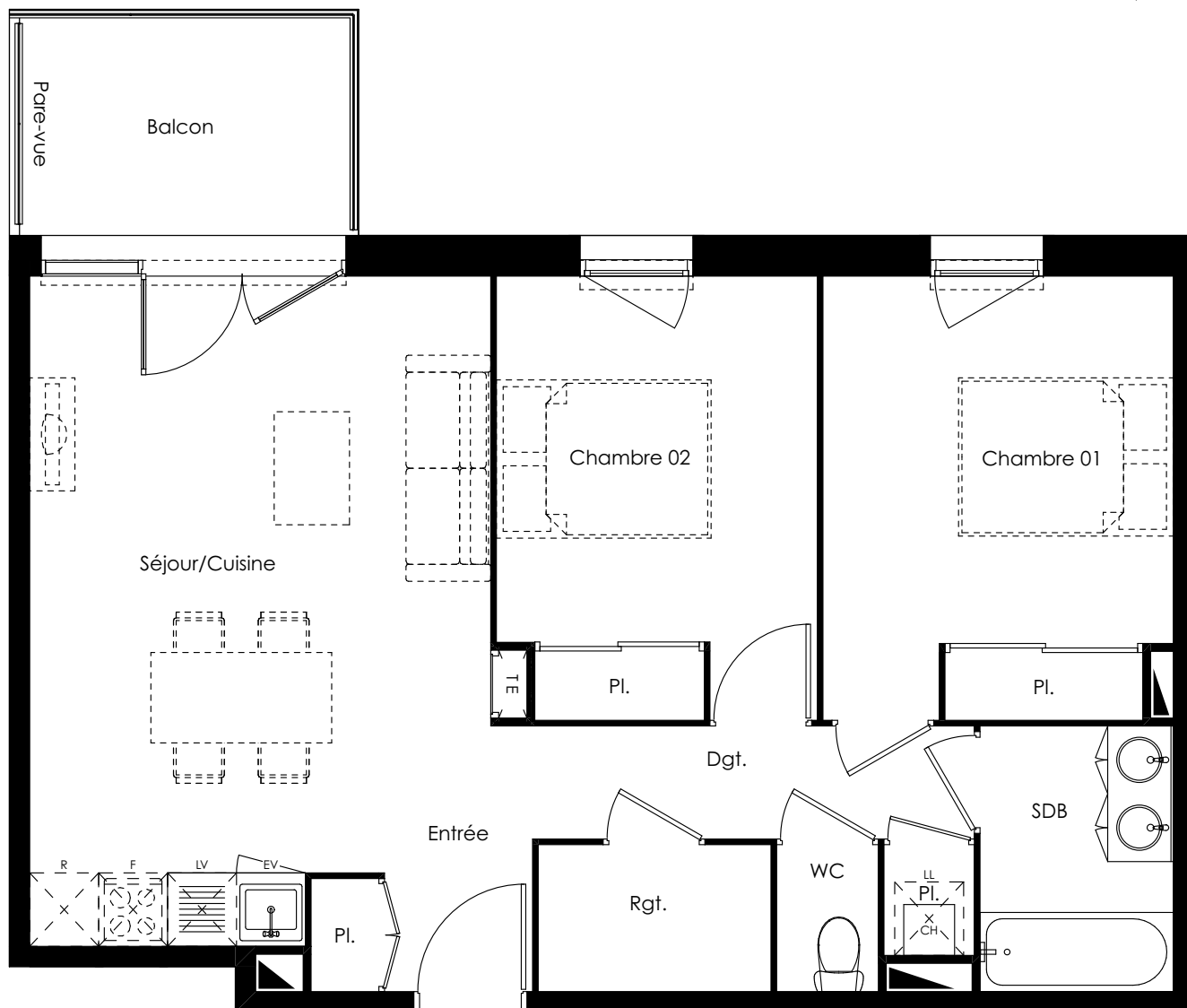
Plan provisoire
