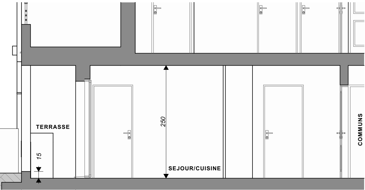
COUPE
