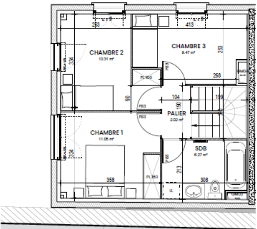
1er étage
