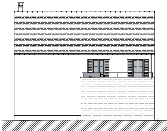
FACADE NORD
