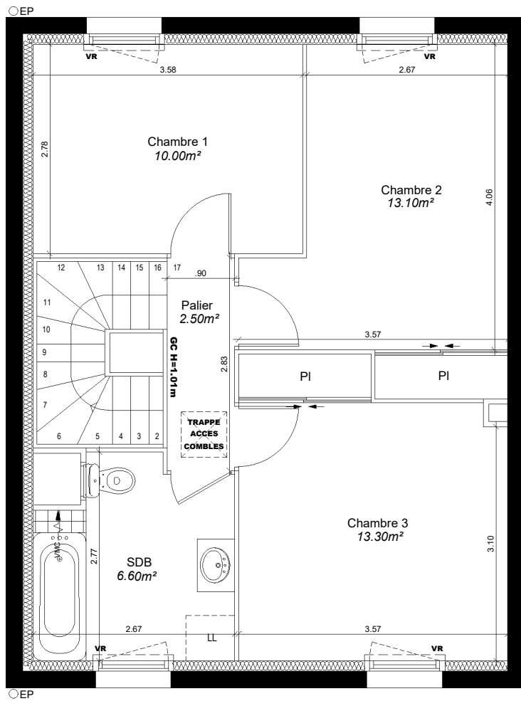
- Niveau 1 -
