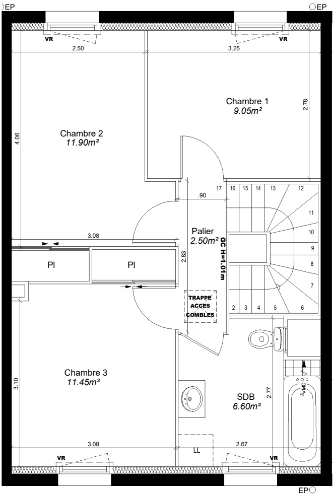
- Niveau 1 -
