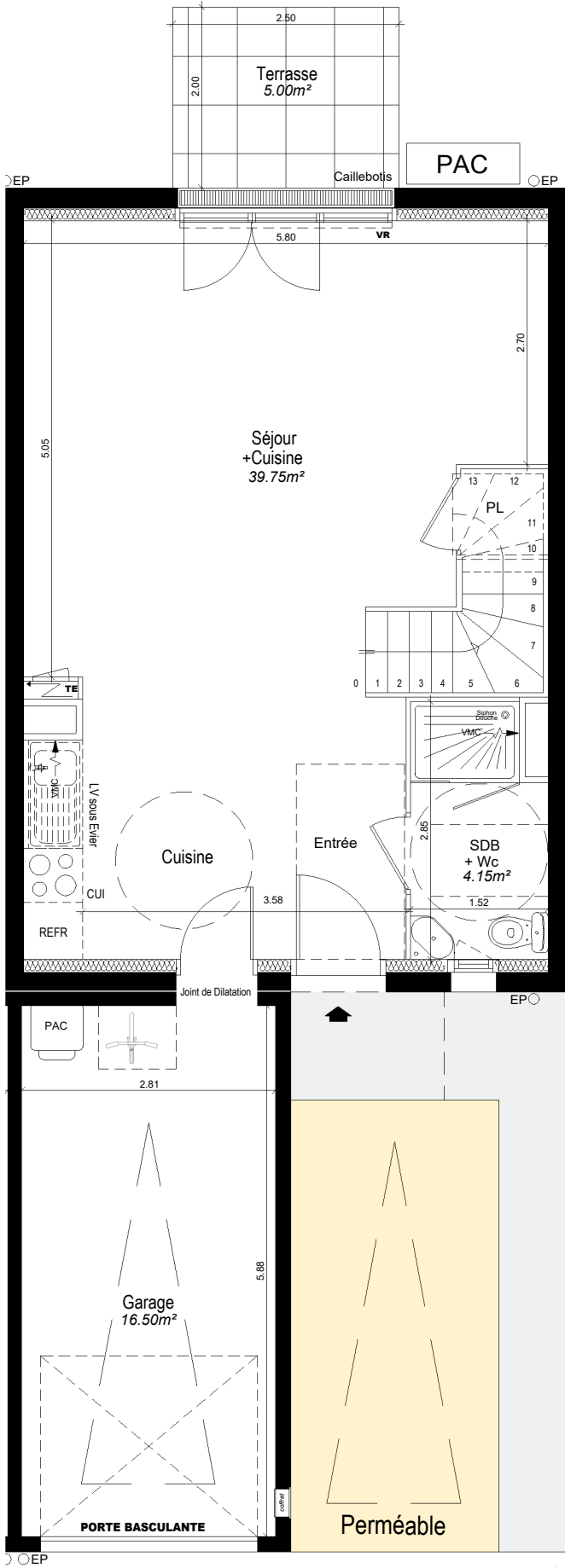
- Niveau Rez-de-chaussée -
