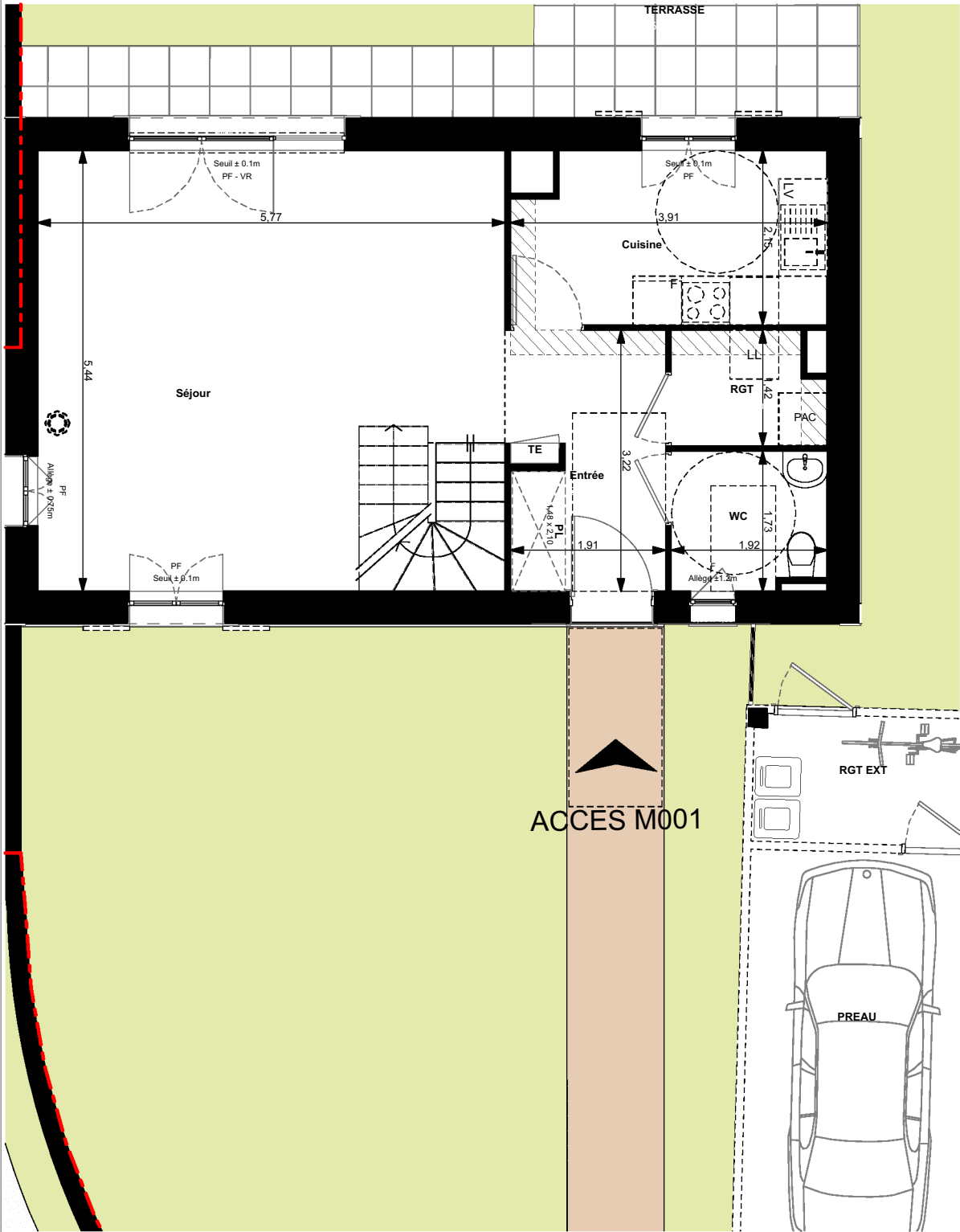
Rez-de-chaussée
