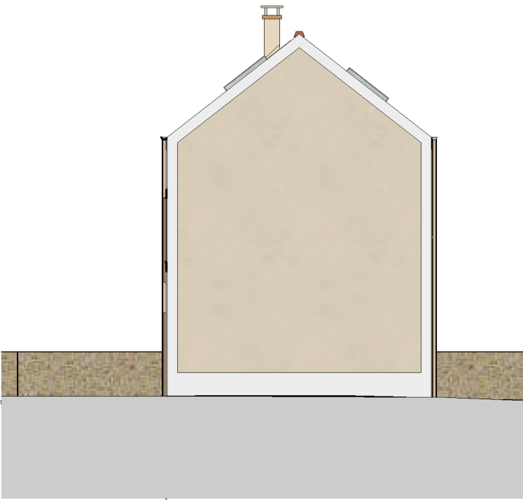
Façade Sud 1:125
