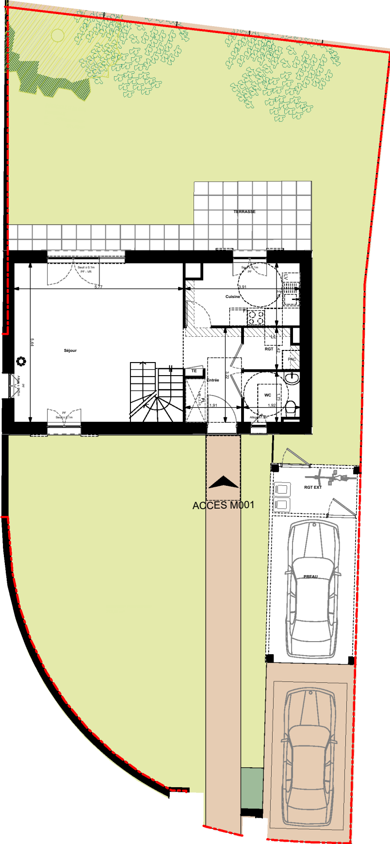
Plan du rez-de-chaussée 1:125
