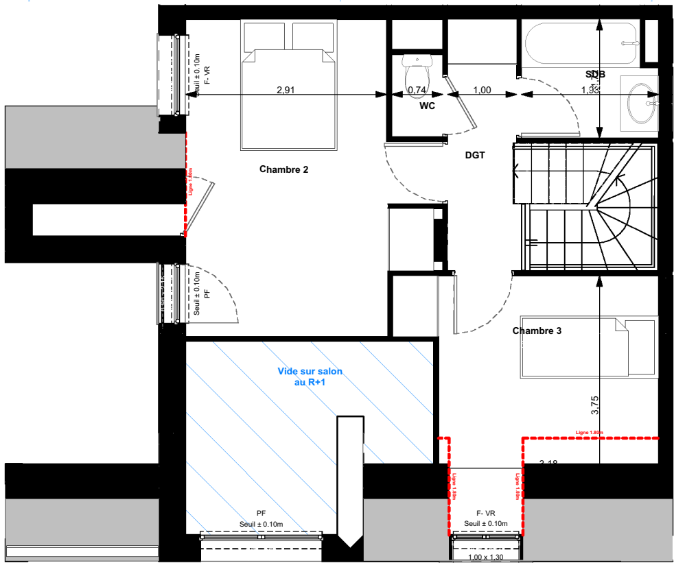
1er étage - Bas duplex 1:75
