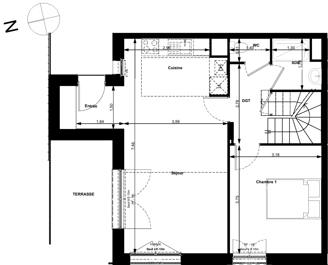
1er étage - Bas duplex 1:75
