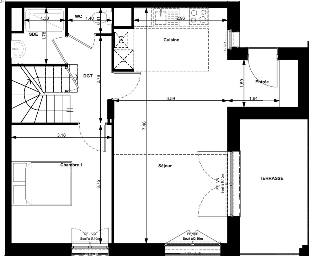
1er étage - Bas duplex 1:75
