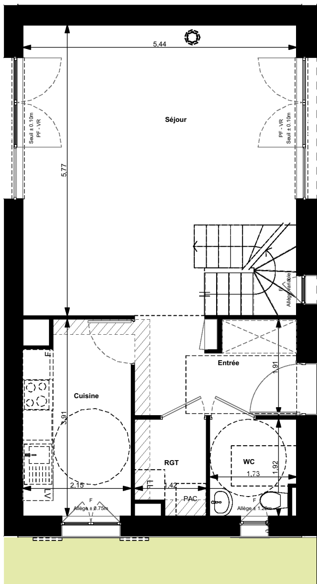
Rez-de-chaussée 1:75
