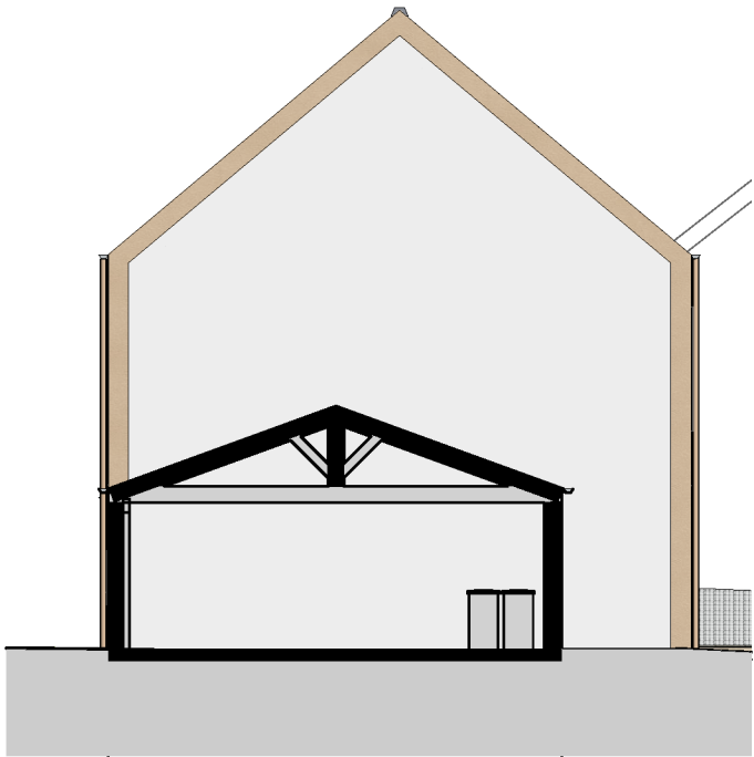
Façade Nord 1:125
