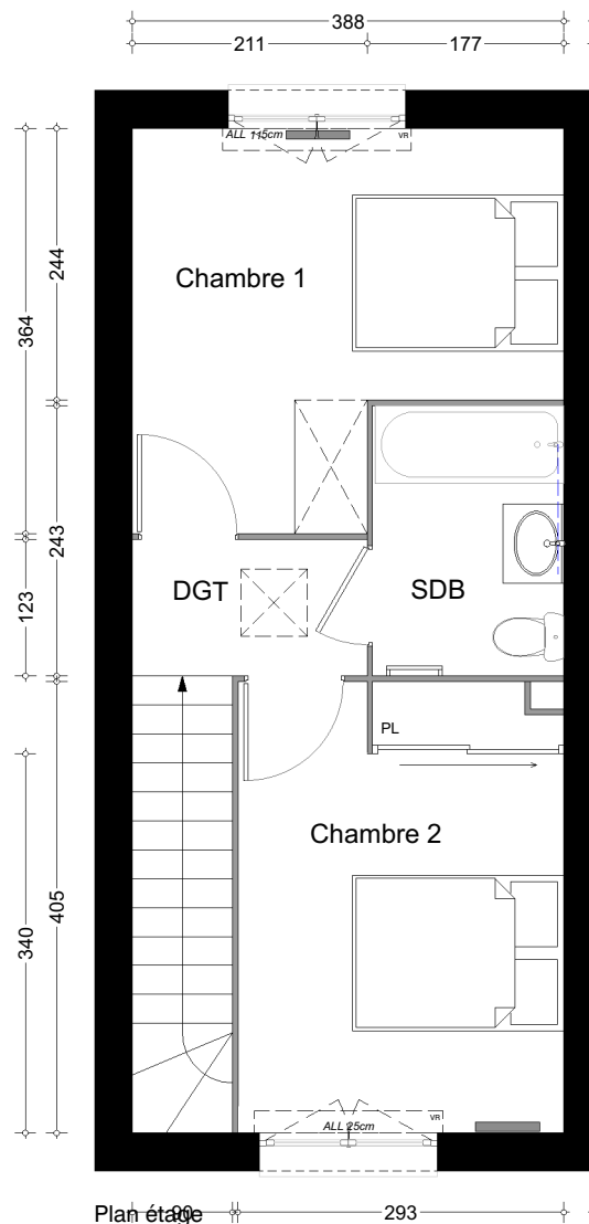
Plan étage
