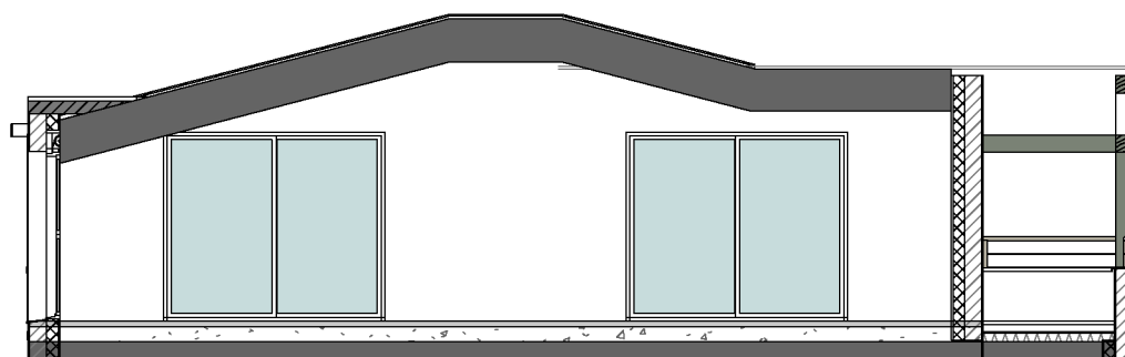
Coupe sur séjour 1206 Ech 1 : 100
