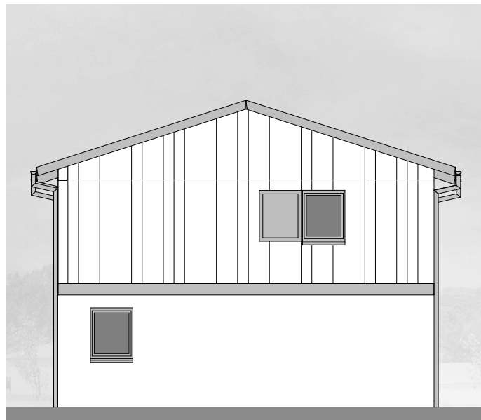
FAÇADE OUEST
