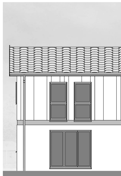
FAÇADE NORD
