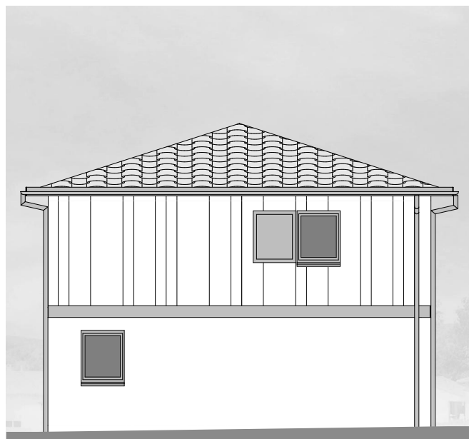
FAÇADE OUEST
