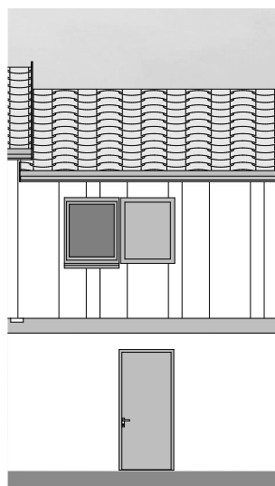
FAÇADE EST
