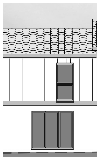
FAÇADE OUEST
