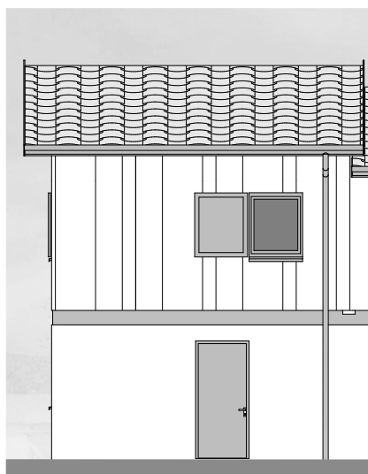
FAÇADE EST
