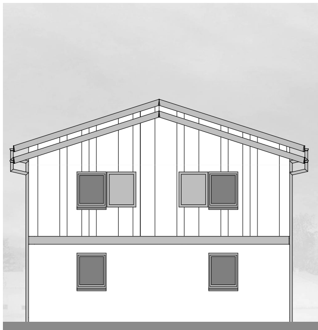
FAÇADE SUD
