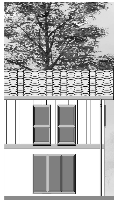
FAÇADE OUEST
