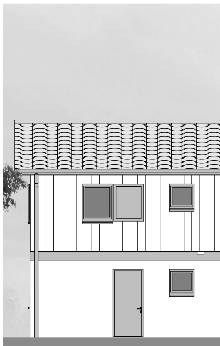
FAÇADE EST
