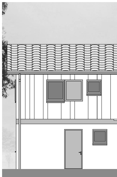
FAÇADE EST
