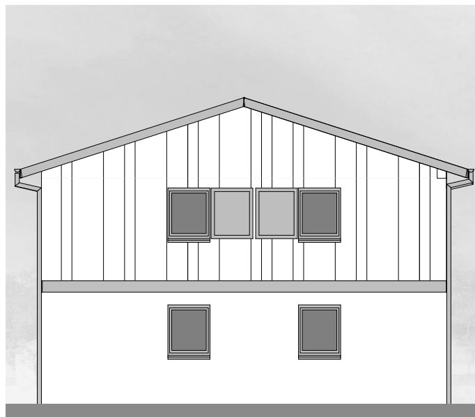
FAÇADE SUD
