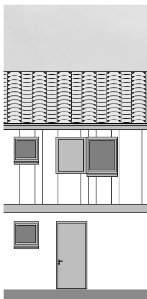
FAÇADE OUEST
