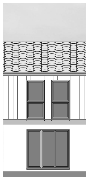
FAÇADE EST
