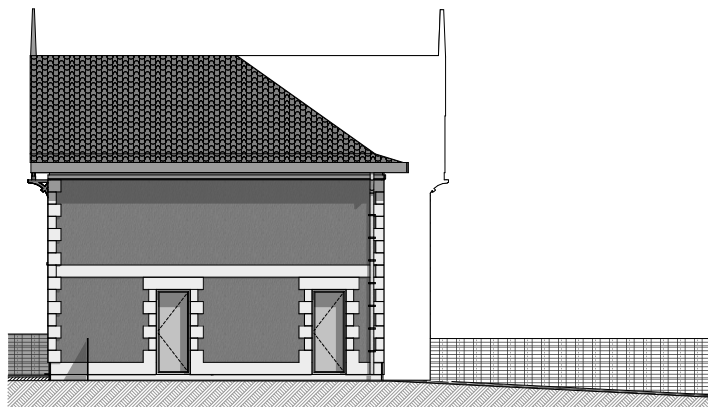
FACADE NORD OUEST
