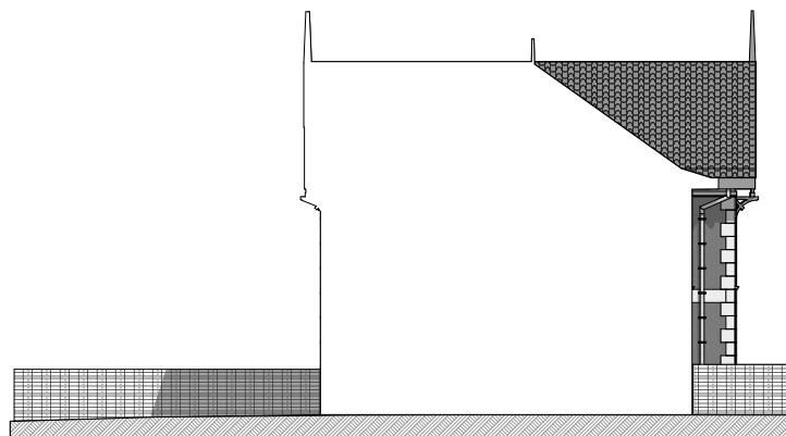
FACADE SUD EST
