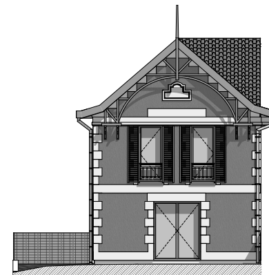
FACADE SUD OUEST
