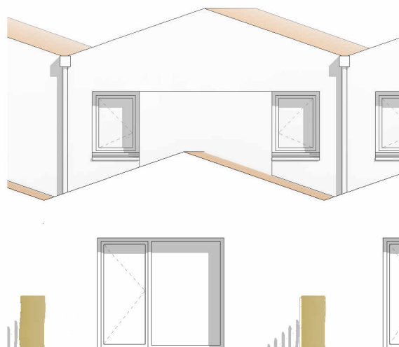
Façade Sud - jardin
