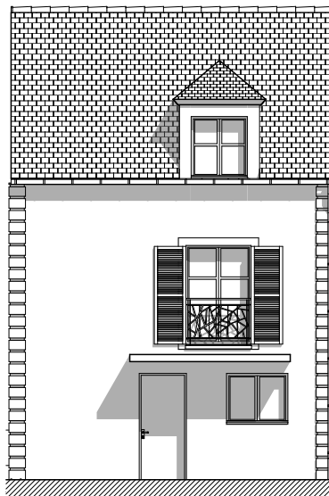
FACADE SUD-EST
