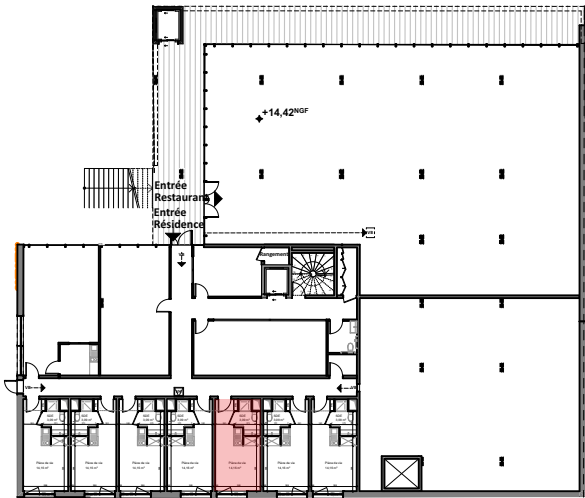
Plan de repérage appartement B-OPEN AIR 203
