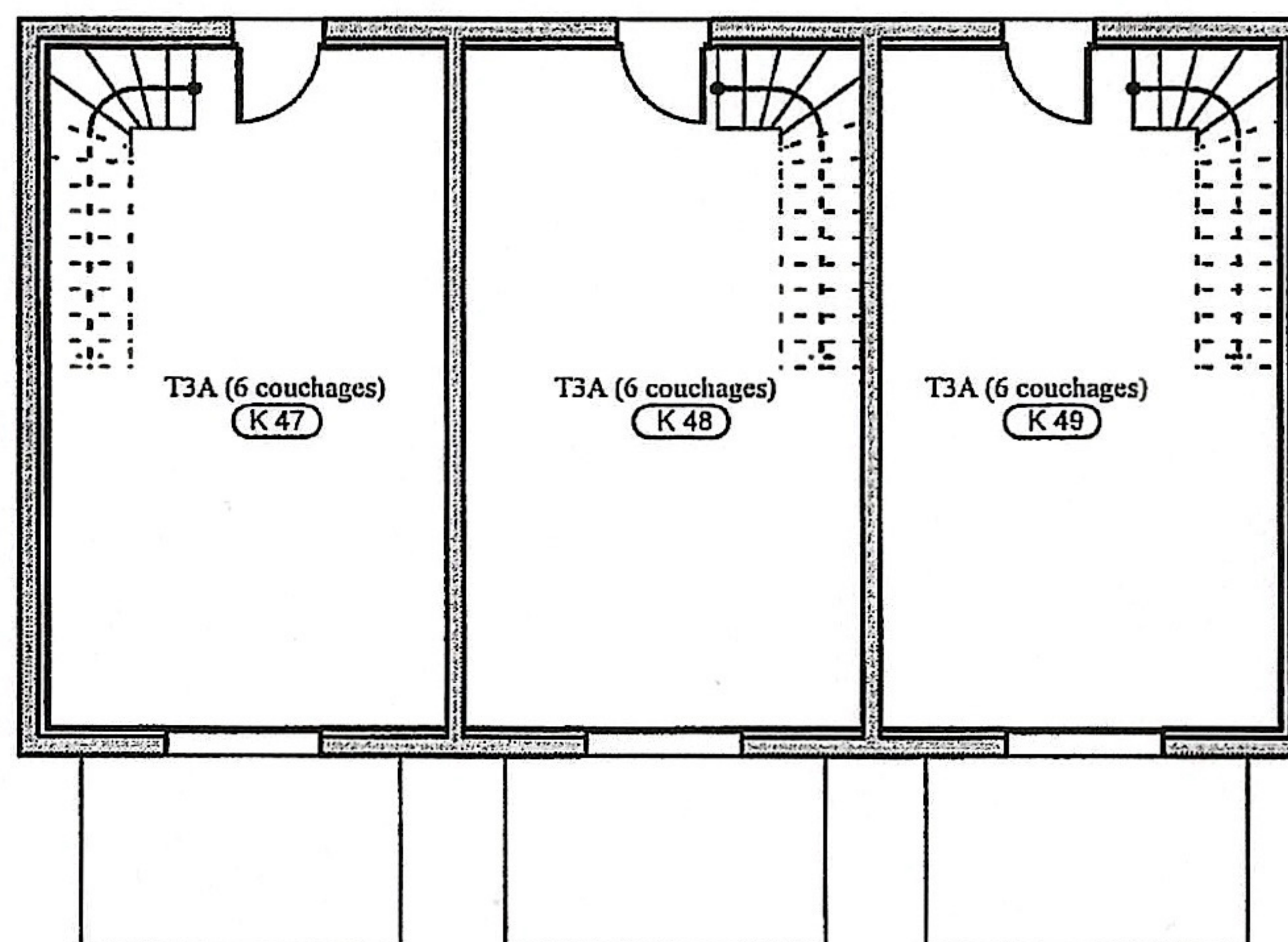
REZ-DE-CHAUSSEE
