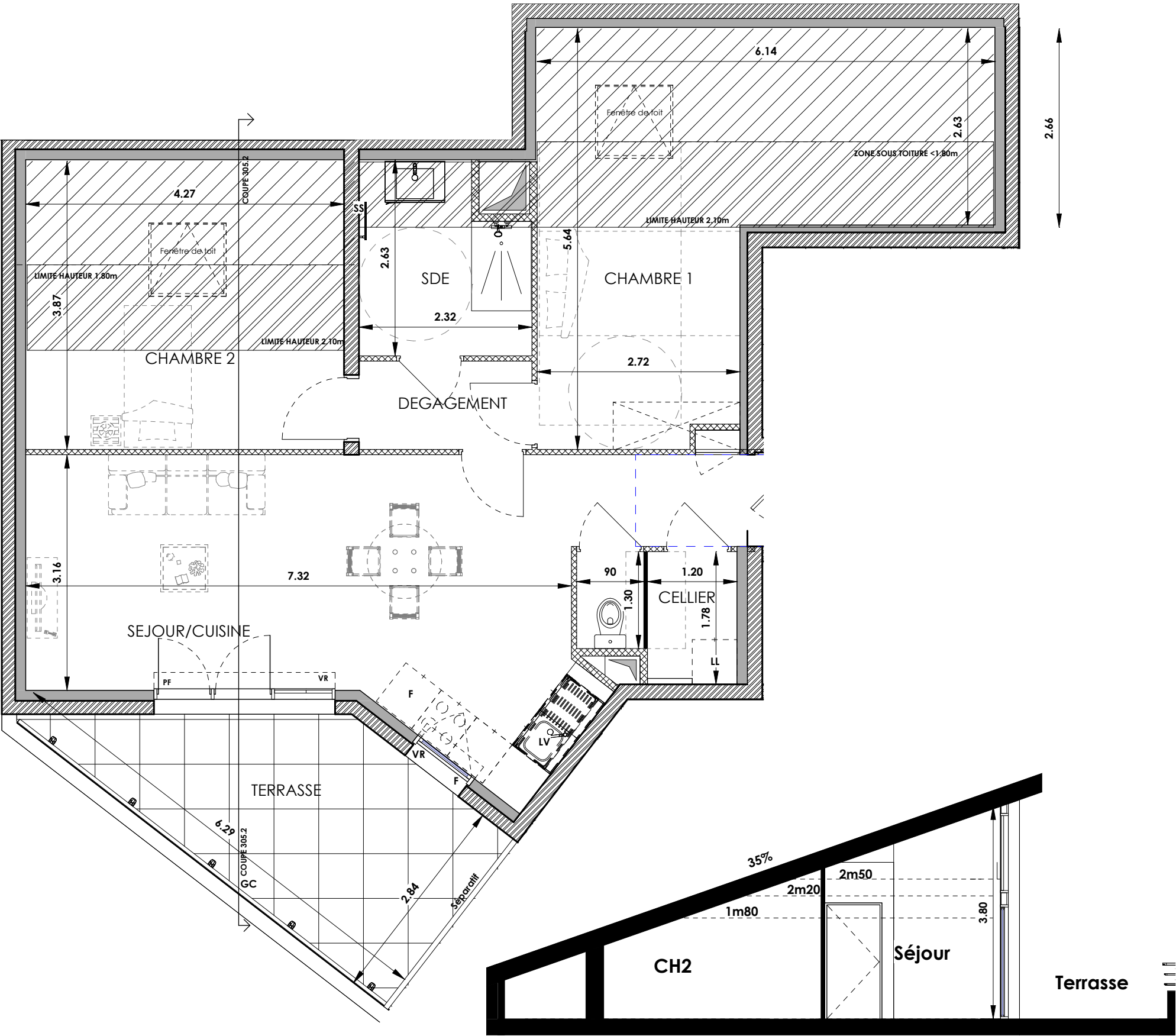
Coupe B305
