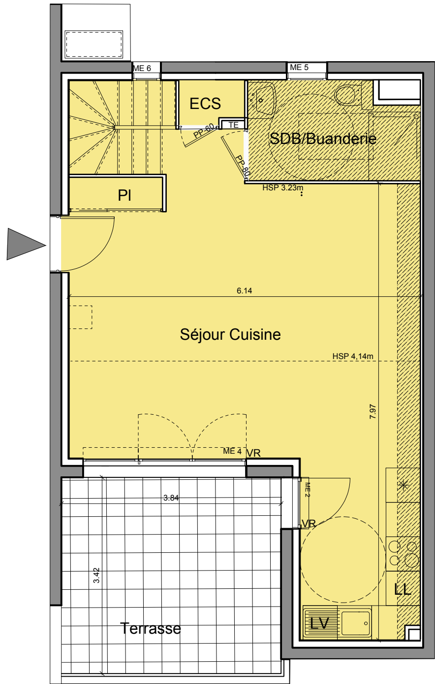
RDC
