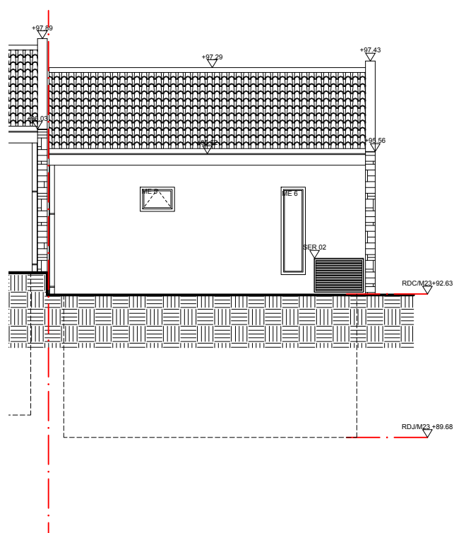
Façade Nord
