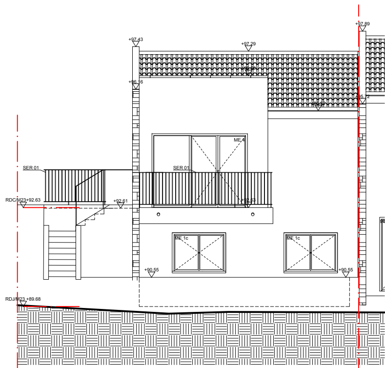
Façade Sud
