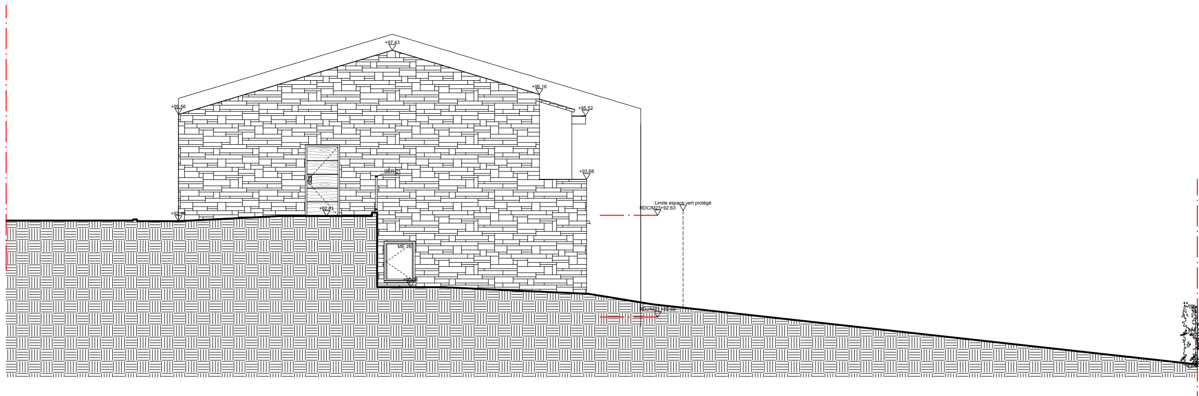
Façade Ouest
