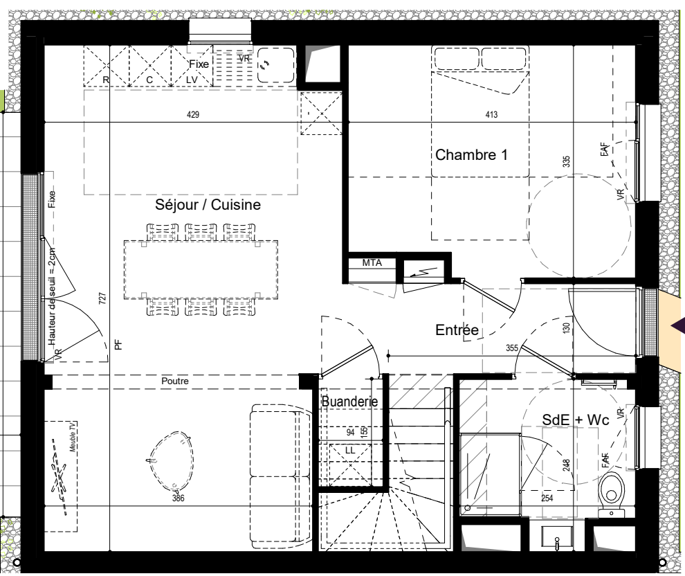
Rez-de-Chaussée
