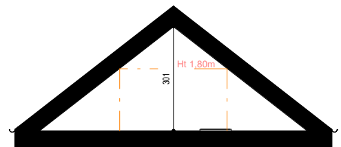
Coupe AA'
