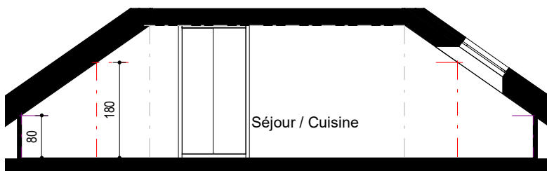
Coupe A
