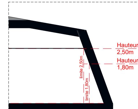
Coupe de principe sur mansarde
